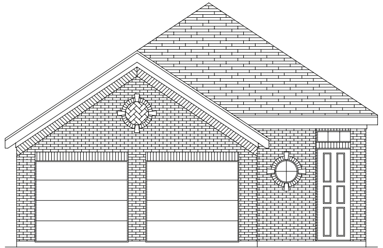
ELEVATION B
