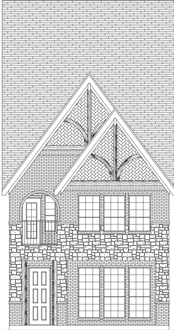
ELEVATION A
