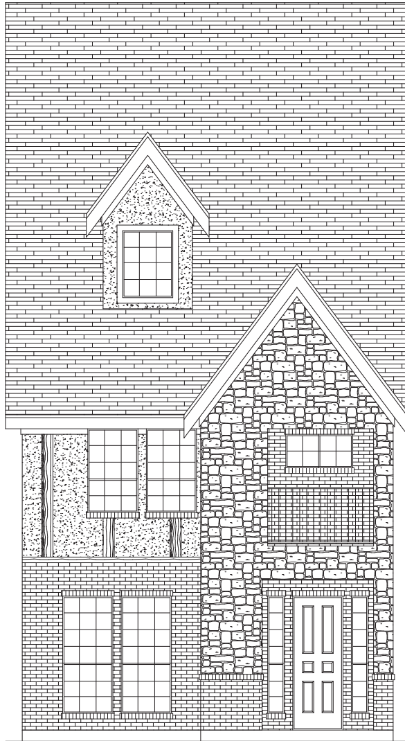
ELEVATION A
