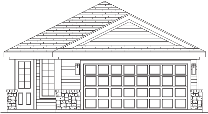
ELEVATION A
