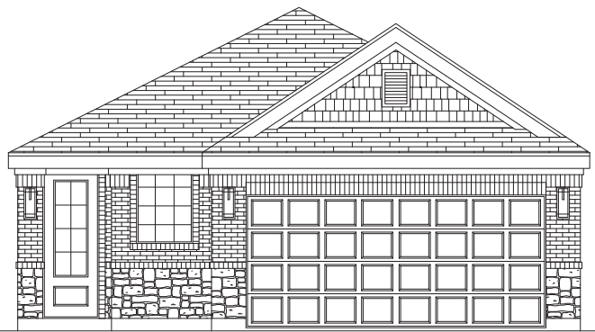
ELEVATION J
