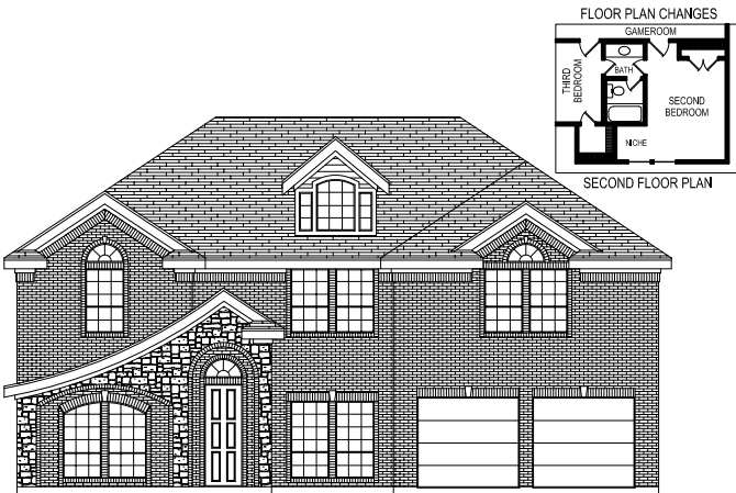
ELEVATION L
